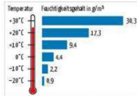
Max. Feuchtigkeitsgehalt in Gramm pro Kubikmeter Luft
